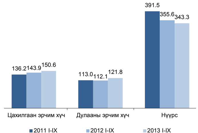
Түлш, эрчим хүчний гол нэр төрлийн бүтээгдэхүүний үйлдвэрлэлийн өөрчлөлт, жил бүрийн эхний 9 сарын байдлаар, хувиар, 2005=100%
