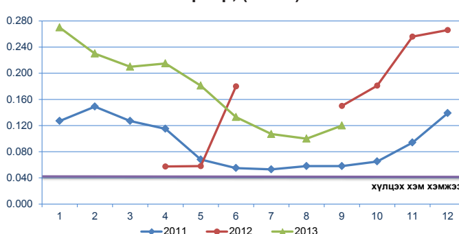
Улаанбаатар хотын Баруун дөрвөн замын орчмын агаар дахь азотын давхар ислийн дундаж агууламж, сараар, (мг/м3)
