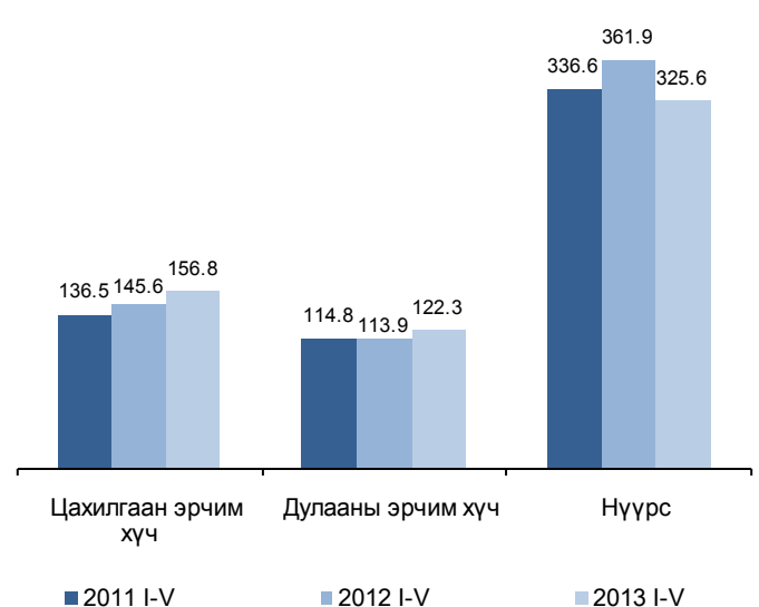
Түлш, эрчим хүчний гол нэр төрлийн бүтээгдэхүүний үйлдвэрлэлийн өөрчлөлт, жил бүрийн эхний 5 сарын байдлаар, хувиар, 2005=100%
