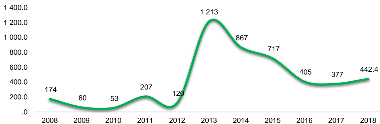
ЗУРАГ 15. АШИГЛАЛТАД ОРУУЛСАН АВТО ЗАМ, км, жил бүрийн эцэст
